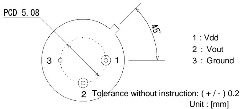
Fig.1 : Dimensions
